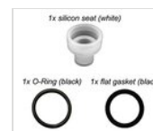
Guarnizioni per tutti rubinetti tranne RUB-ECO GUARNIZIONI SET
